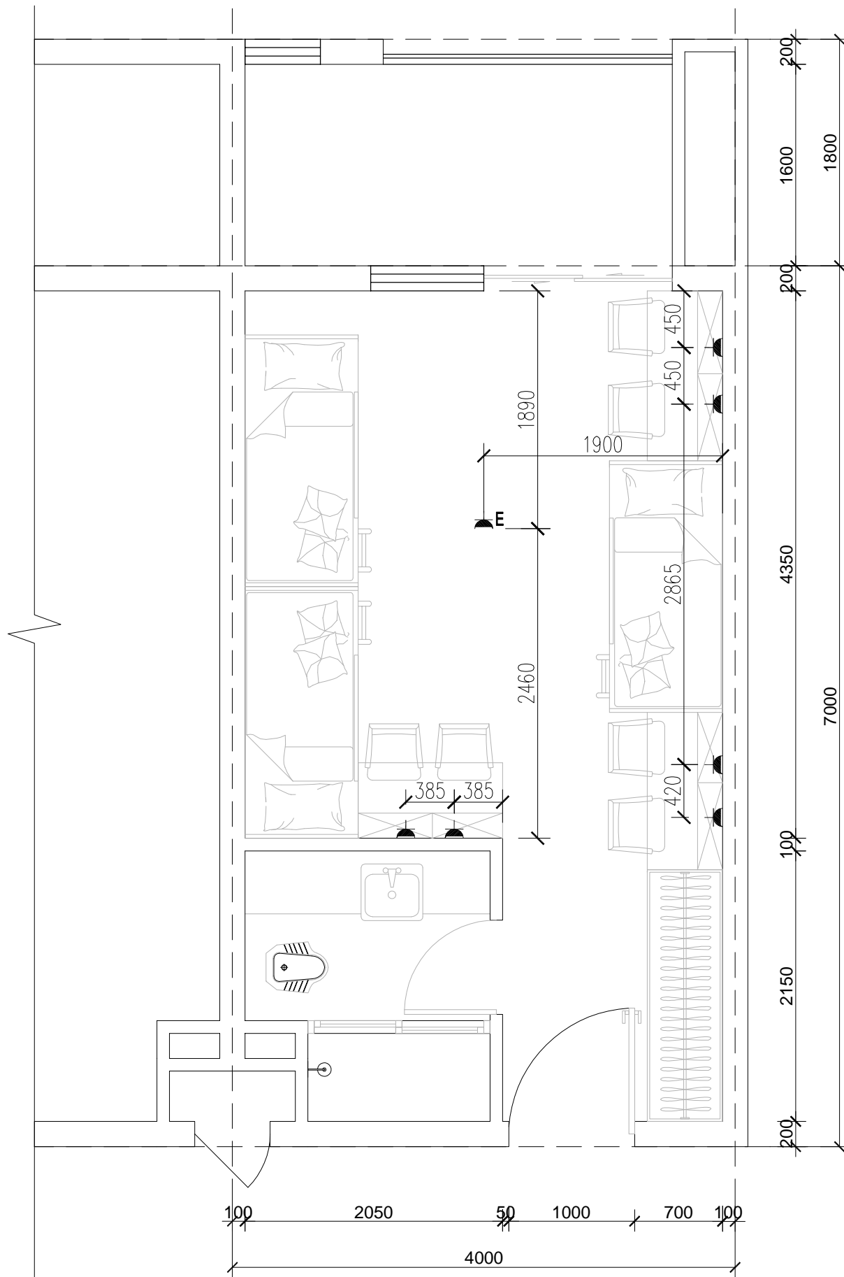
1-5 PLAN 插座布置图 Scale: 1:40
