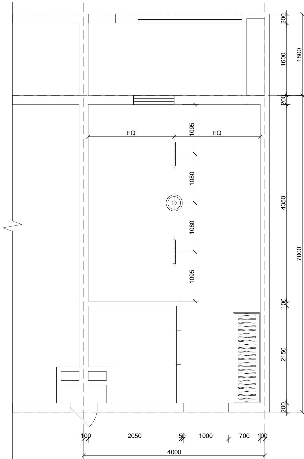
1-3 PLAN 天花灯具定位图 Scale: 1:40
