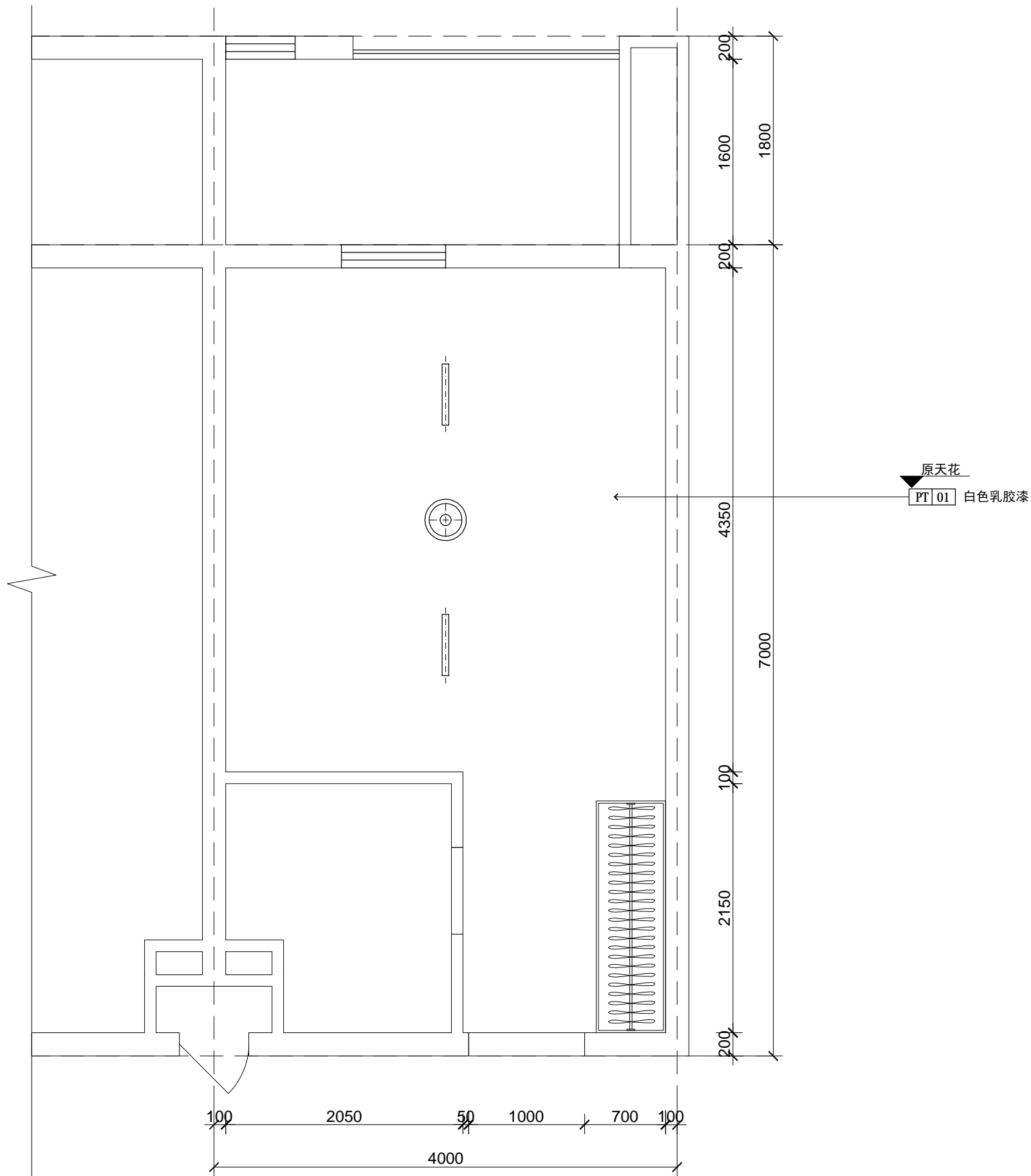
1-2 PLAN 天花布置图 Scale: 1:40
