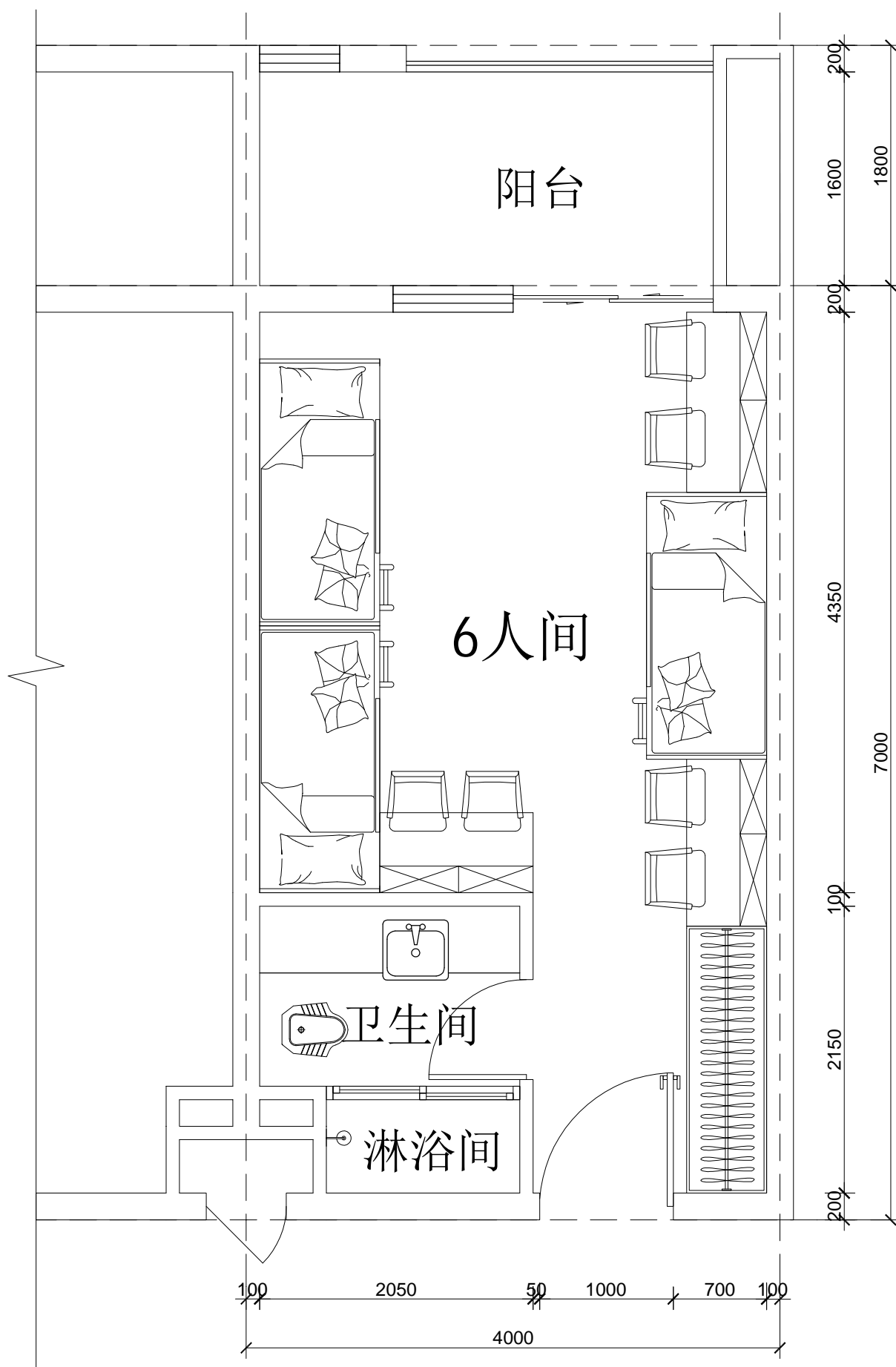
1-1 PLAN 平面布置图 Scale: 1:40
