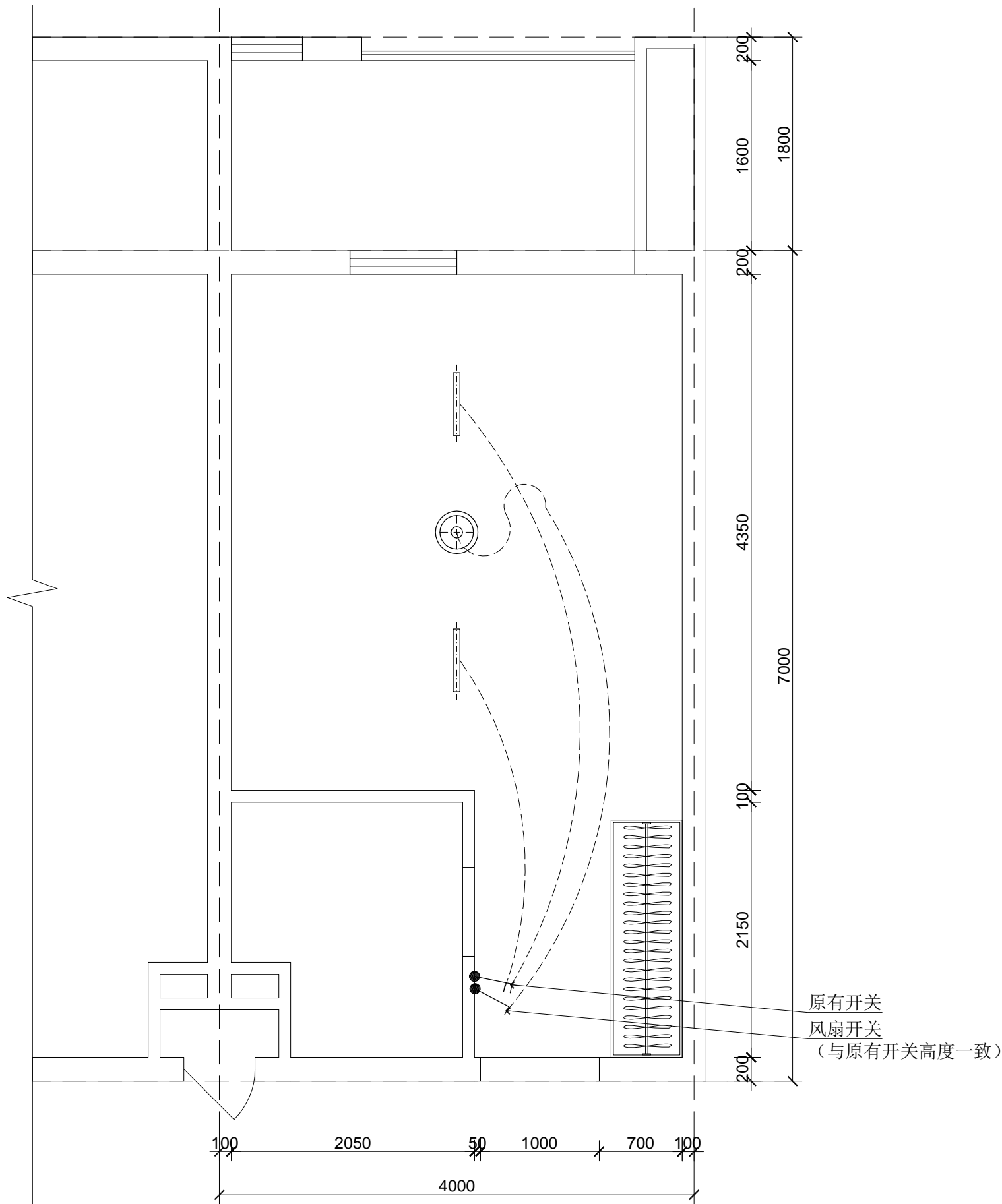
1-4 PLAN 天花灯具连线图 Scale: 1:40
